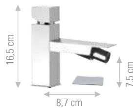
CU604 Monocomando bidet, con scarico. Single-lever bidet mixer, with pop-up waste.
