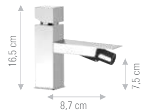
CU604B Monocomando bidet, senza scarico. Single-lever bidet mixer, without waste.
